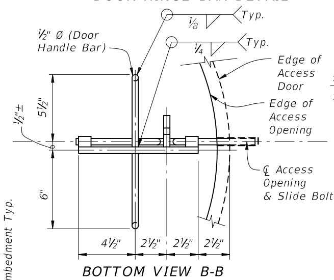
DOOR HINGE BAR DETAIL
