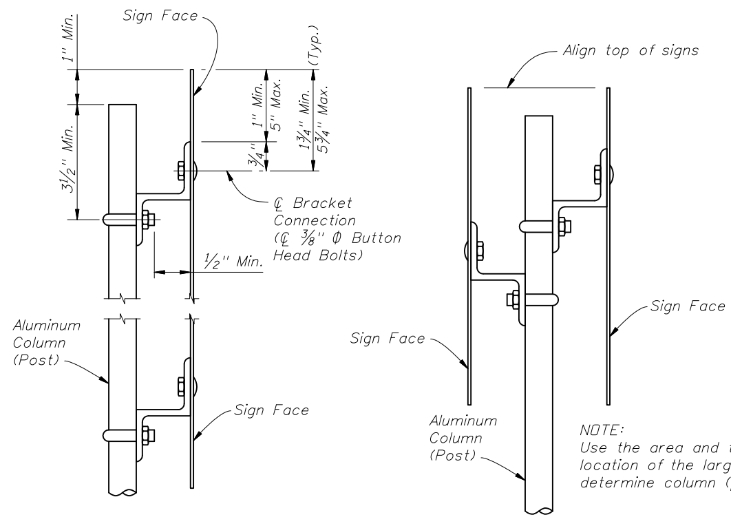
VIEW A-A
