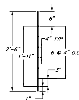
F 2 SECTION BACKING PANEL N.T.S.
