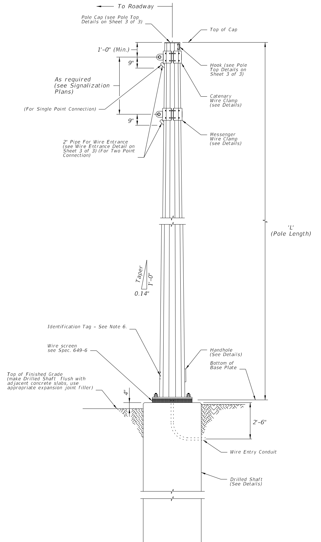
ELEVATION
